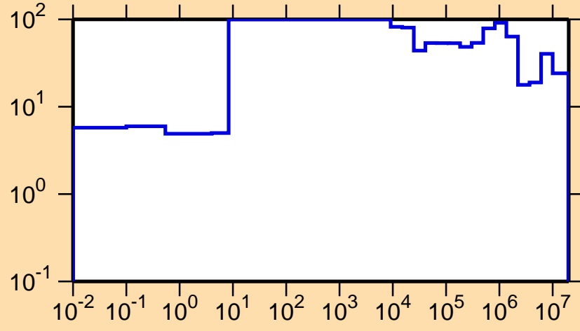
\Delta\sigma/\sigma vs. E for ^{254}\text{Lw}(n,el.)
