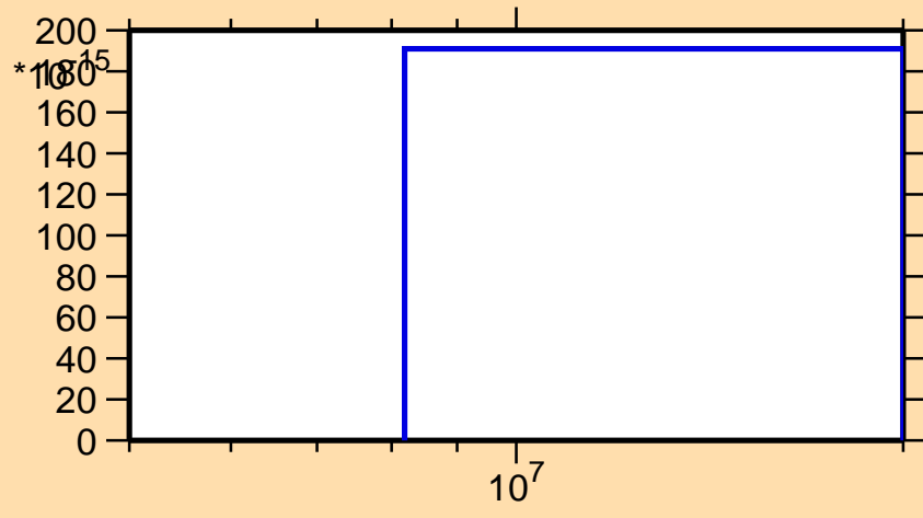
\sigma vs. E for ^{254}\text{Lw}(\text{mt } 45)
