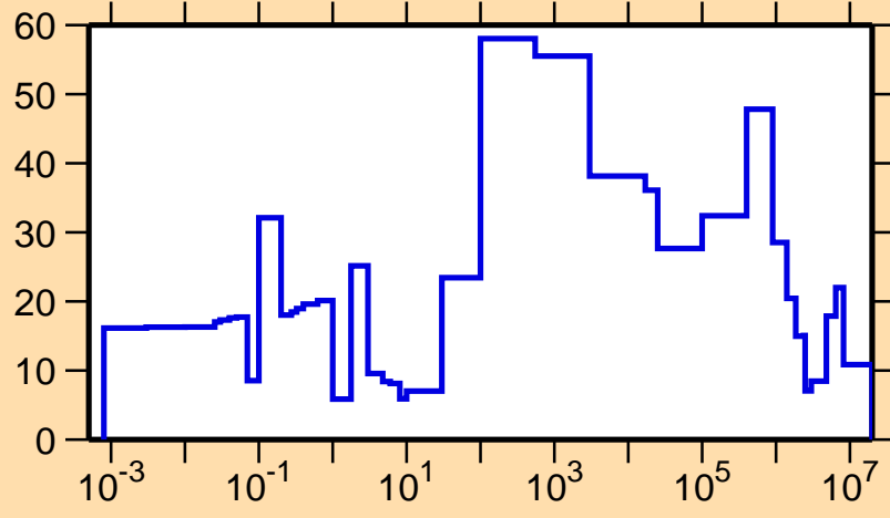
\Delta\sigma/\sigma vs. E for ^{257}\text{Lw}(n,el.)
