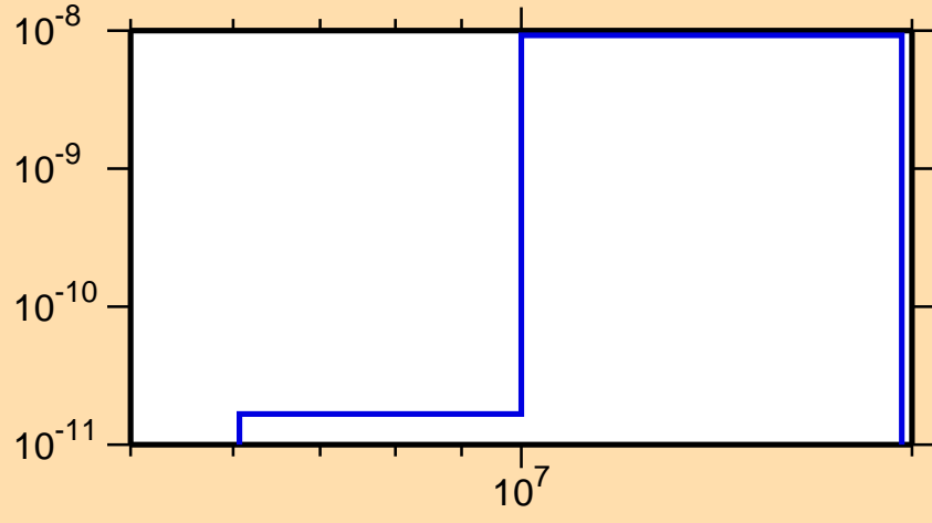
\sigma vs. E for ^{248}\text{Md}(\text{mt } 45)
