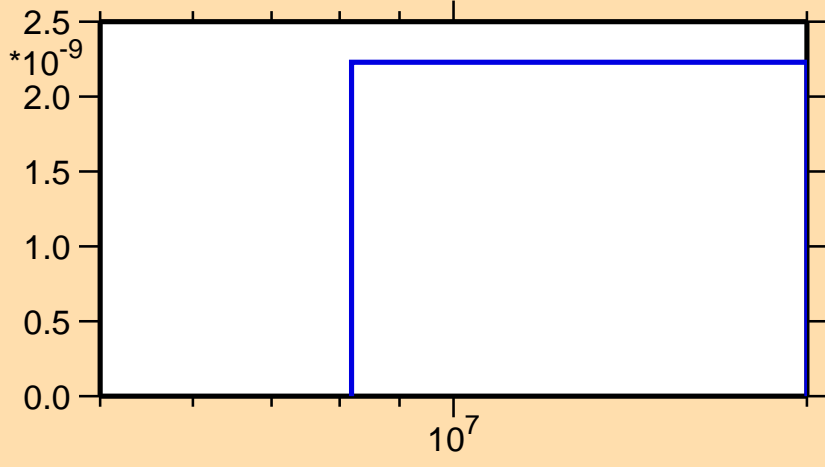
\sigma vs. E for ^{85}\text{Mo}(\text{mt } 34)
