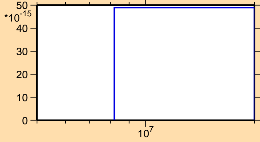
\sigma vs. E for ^{86}\text{Mo} (mt 34)
