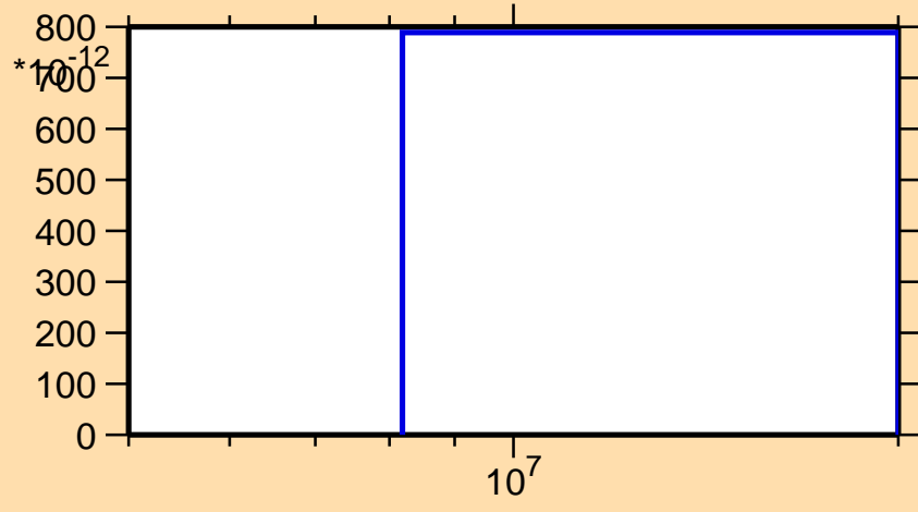
\sigma vs. E for ^{86}\text{Mo}(\text{mt } 45)
