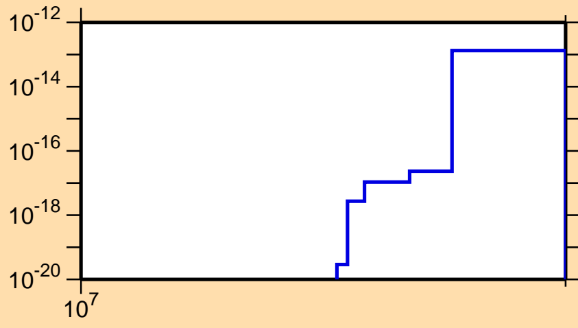
\sigma vs. E for ^{88}\text{Mo} (mt 34)
