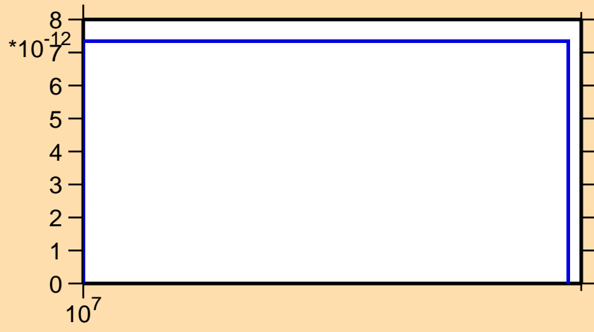
\sigma vs. E for ^{88}\text{Mo} (mt 45)
