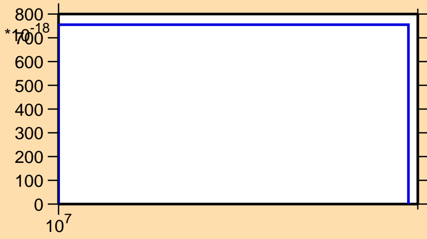
\sigma vs. E for ^{88}\text{Mo}(\text{mt } 34)
