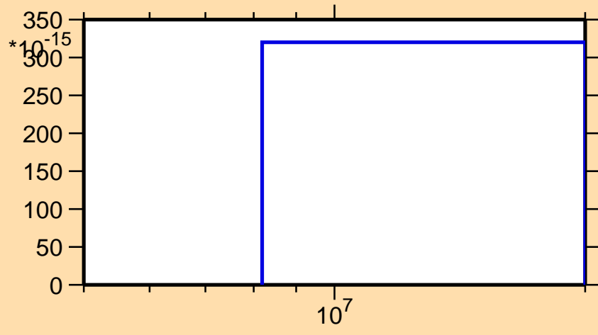
\sigma vs. E for ^{88}\text{Nb}(\text{mt } 34)
