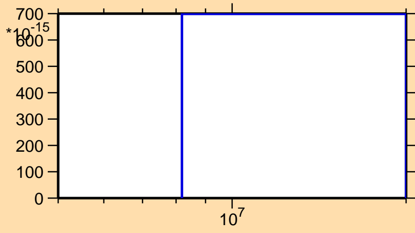
\sigma vs. E for ^{253}\text{No}(\text{mt } 34)
