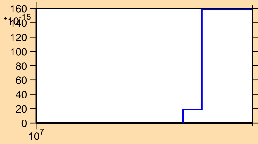
\sigma vs. E for ^{254}\text{No}(\text{mt } 45)
