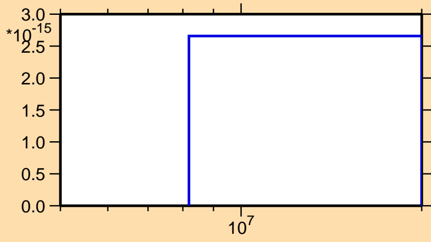
\sigma vs. E for ^{254}\text{No}(\text{mt } 45)
