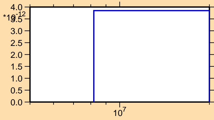
\sigma vs. E for ^{177}\text{Os} (mt 34)
