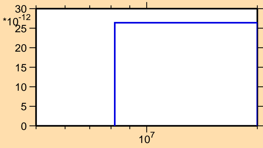
\sigma vs. E for ^{226}\text{Pa}(\text{mt } 45)
