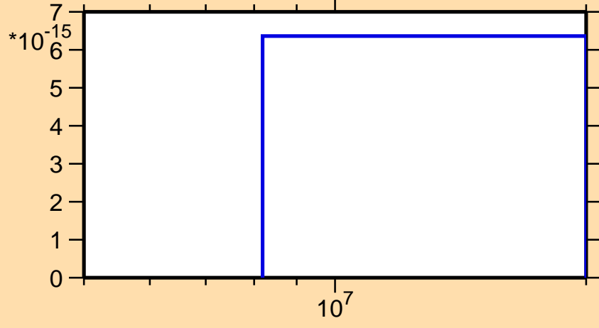
\sigma vs. E for ^{226}\text{Pa}(\text{mt } 34)
