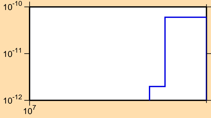
\sigma vs. E for ^{196}\text{Po}(\text{mt } 34)
