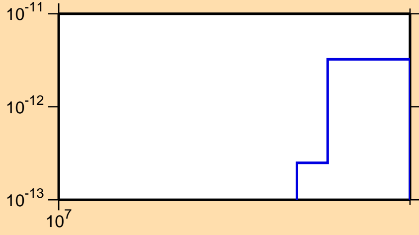
\sigma vs. E for ^{206}\text{Po}(\text{mt } 45)
