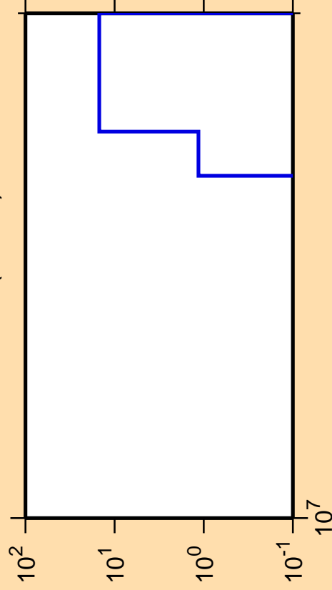
\Delta\sigma/\sigma vs. E for ^{206}\text{Po}(\text{mt } 45)
