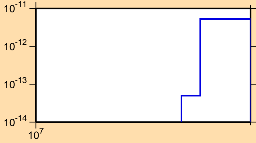
\sigma vs. E for ^{209}\text{Po}(\text{mt } 34)
