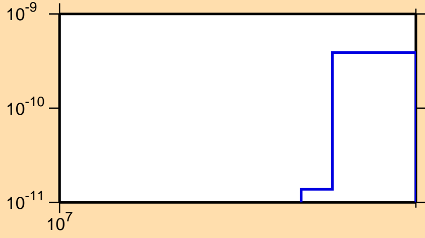
\sigma vs. E for ^{183}\text{Pt}(\text{mt } 34)
