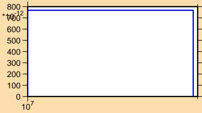
\sigma vs. E for ^{183}\text{Pt}(\text{mt } 45)
