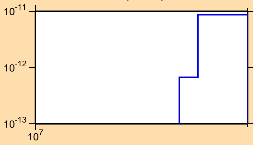
\sigma vs. E for ^{189}\text{Pt}(\text{mt } 45)
