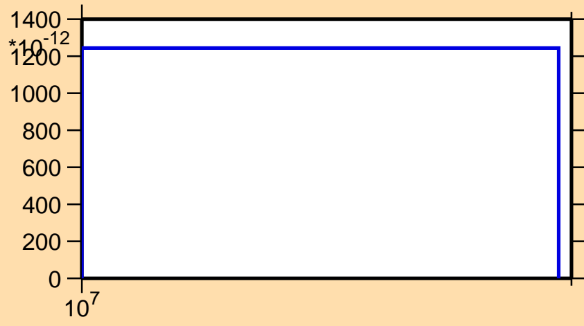
\sigma vs. E for ^{166}\text{Re}(\text{mt } 34)
