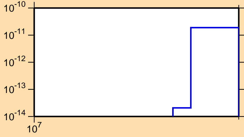
\sigma vs. E for ^{111}\text{Sn}(\text{mt } 45)
