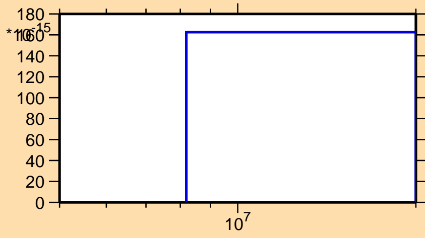
\sigma vs. E for ^{111}\text{Sn}(\text{mt } 34)
