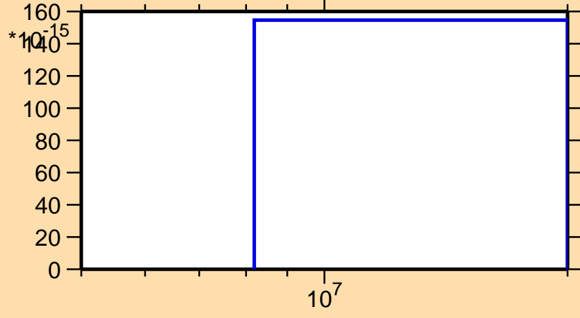
\sigma vs. E for ^{111}\text{Sn}(\text{mt } 45)
