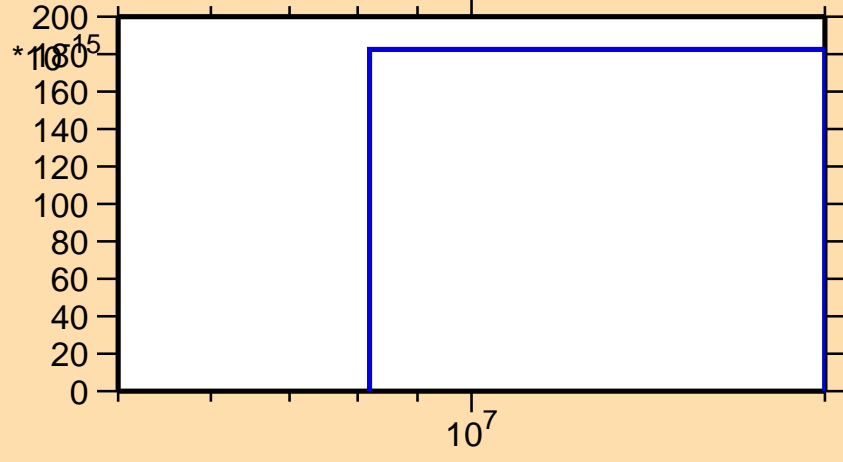
\sigma vs. E for ^{177}\text{Ta}(\text{mt } 45)
